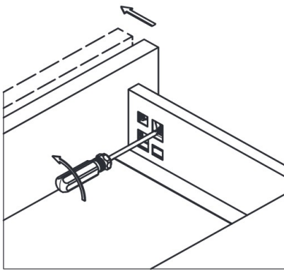
vyjmutí čela zásuvky
