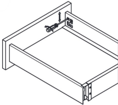
seřízení zásuvky vertikálně (nahoru, dolů)
